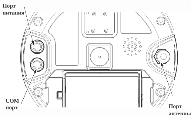
Рис. 1-4. Порты приемника GRX2
