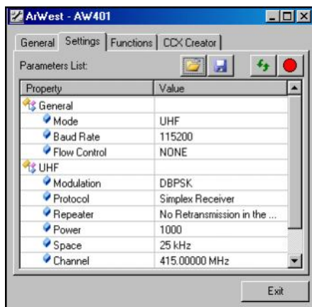
Рис. 3-7. Настройки радиомодема
