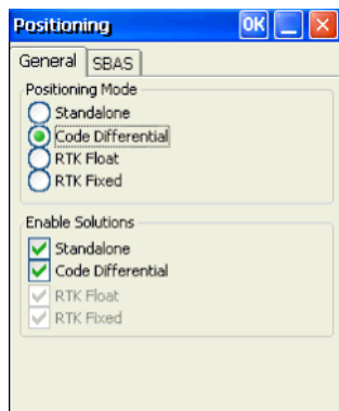
Рис. 3-16. Настройка ровера
