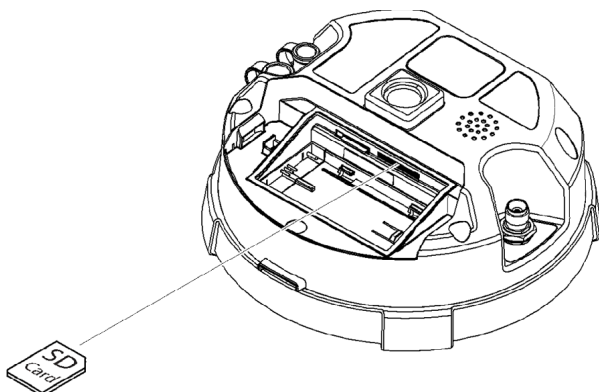
Рис. 2-2. Установка карты SD/SDHC
