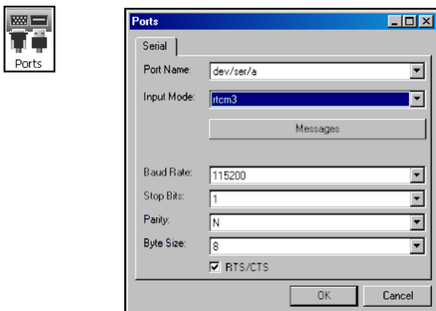
Рис. 3-17. Настройка портов
