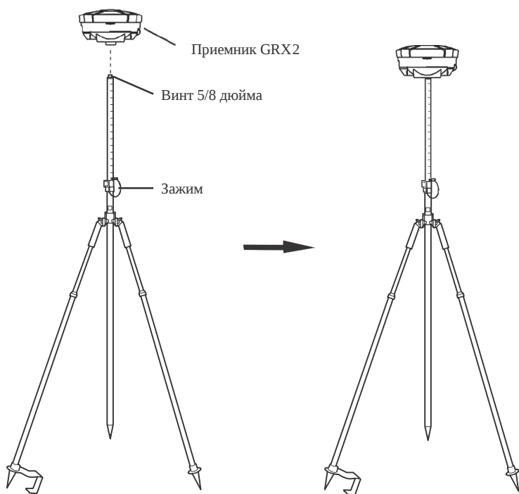
Рис. 4-2. Крепление GRX2 на вешке к биподу
