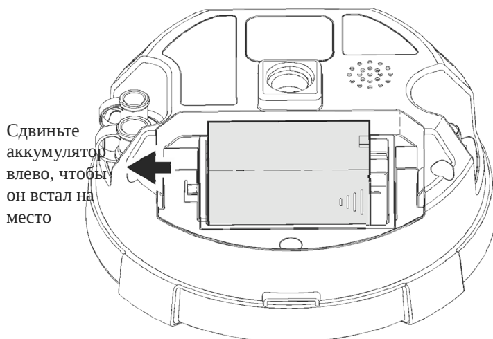
Рис. 2-6. Снимите крышку аккумуляторного отсека
