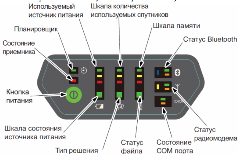
Рис. 1-3. Индикаторная панель GRX2
